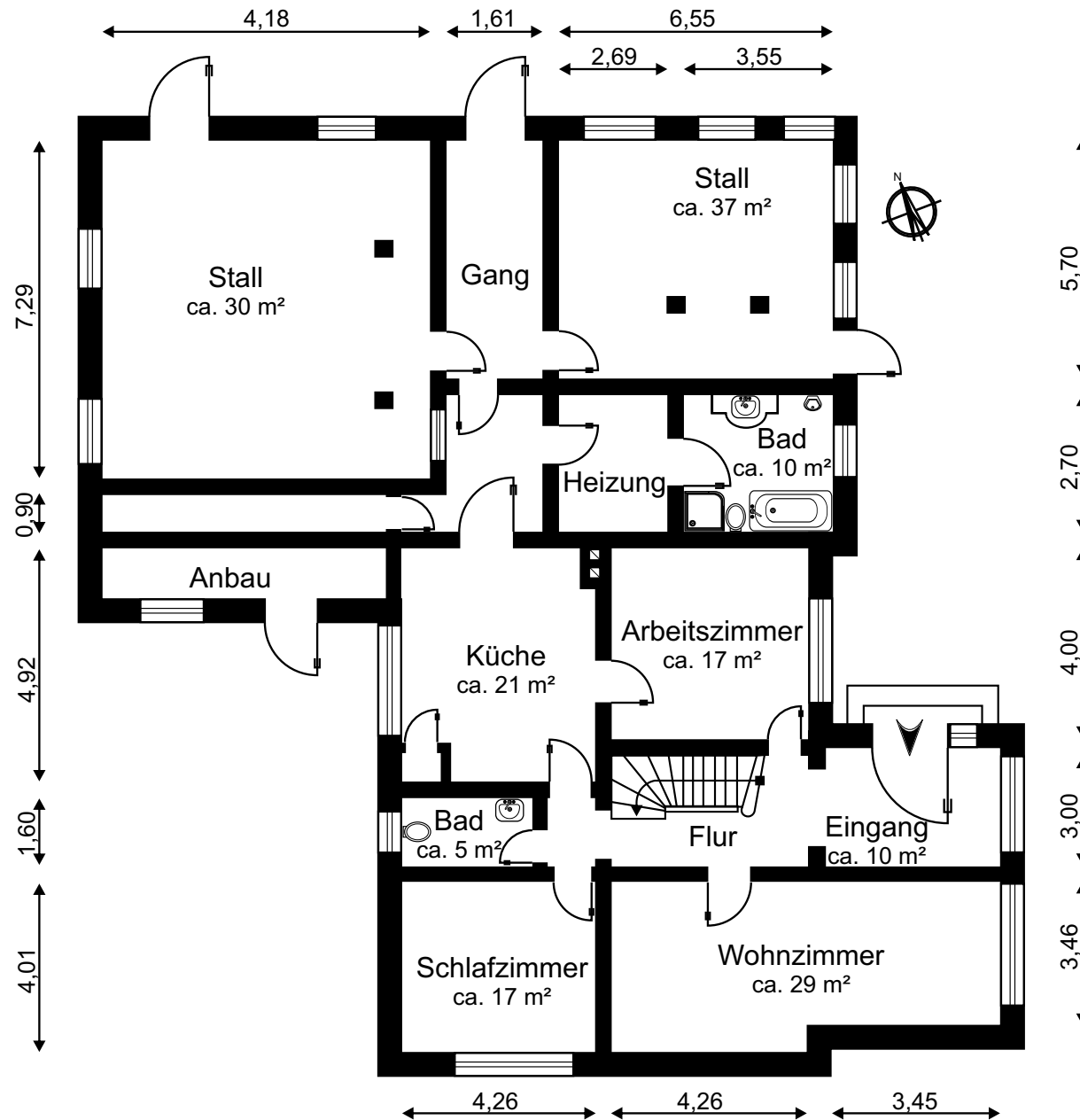
MB 21167 Grundriss Erdgeschoss
