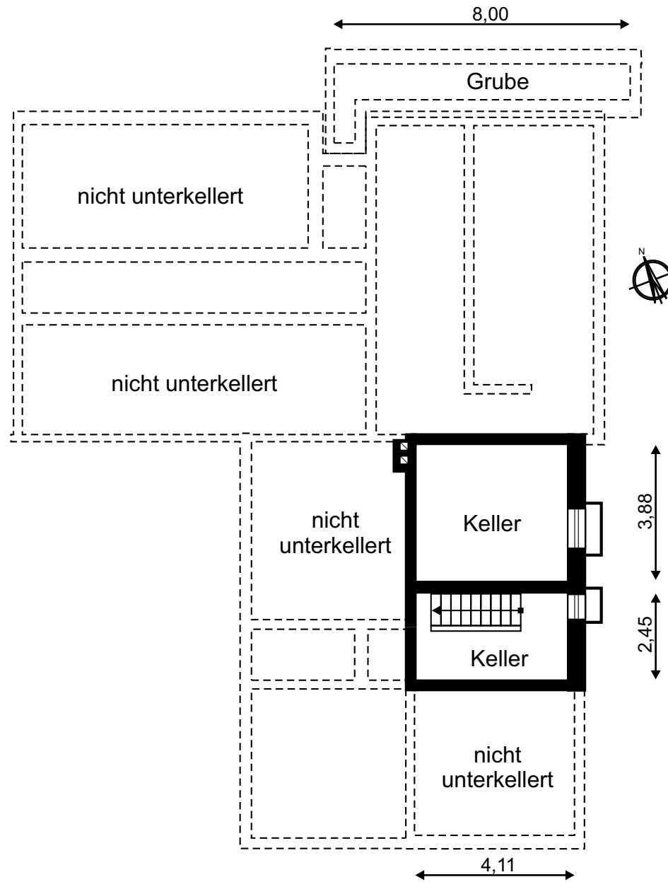
MB 21167 Grundriss Fundamente Grube und Keller
