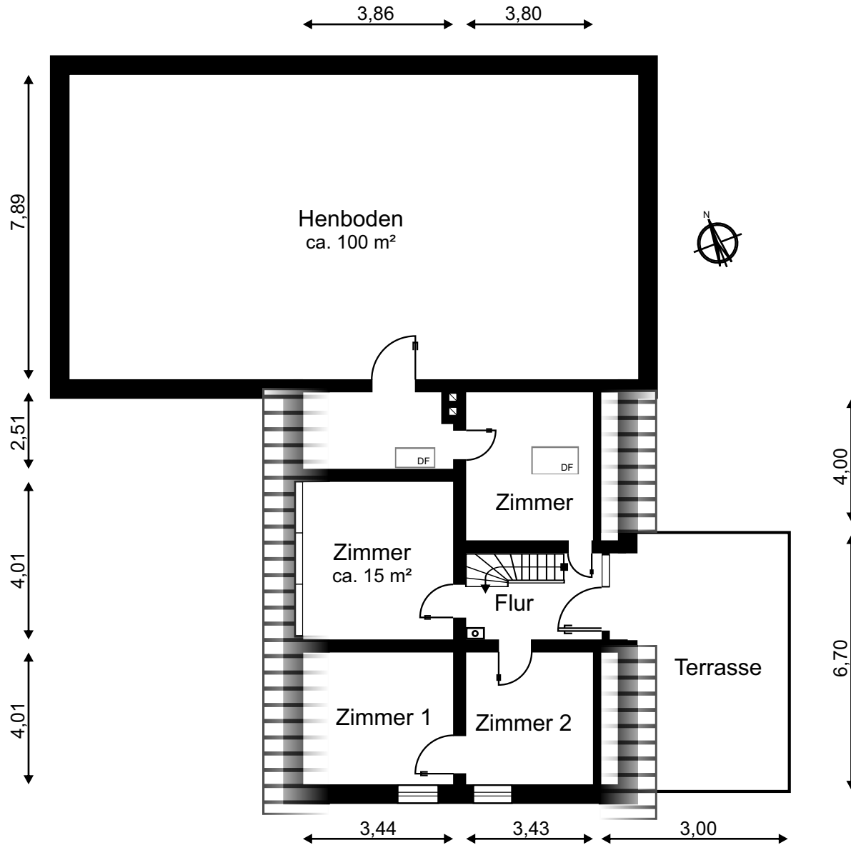
MB 21167 Grundriss Obergeschoss
