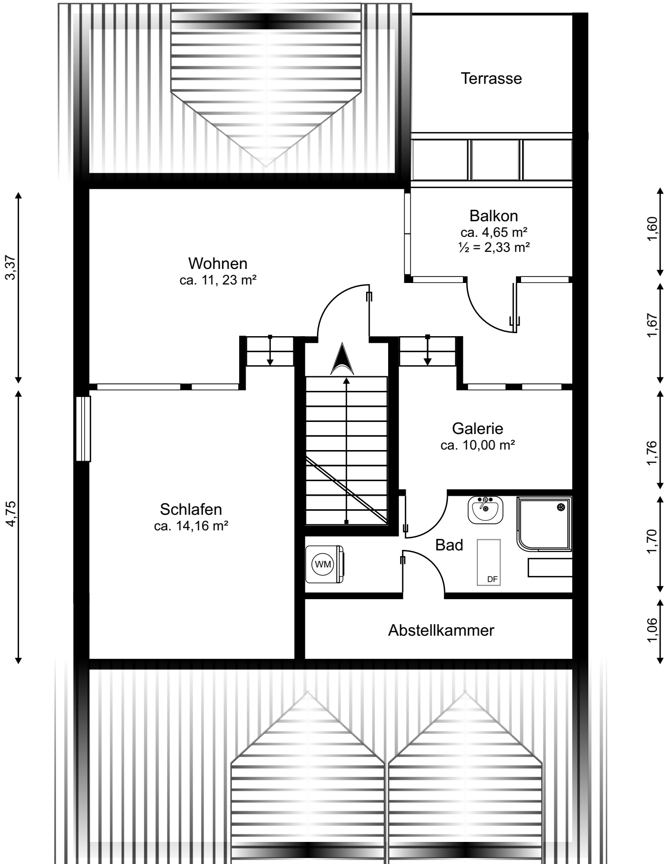
Dachgeschoss Grundriss MB 24207
