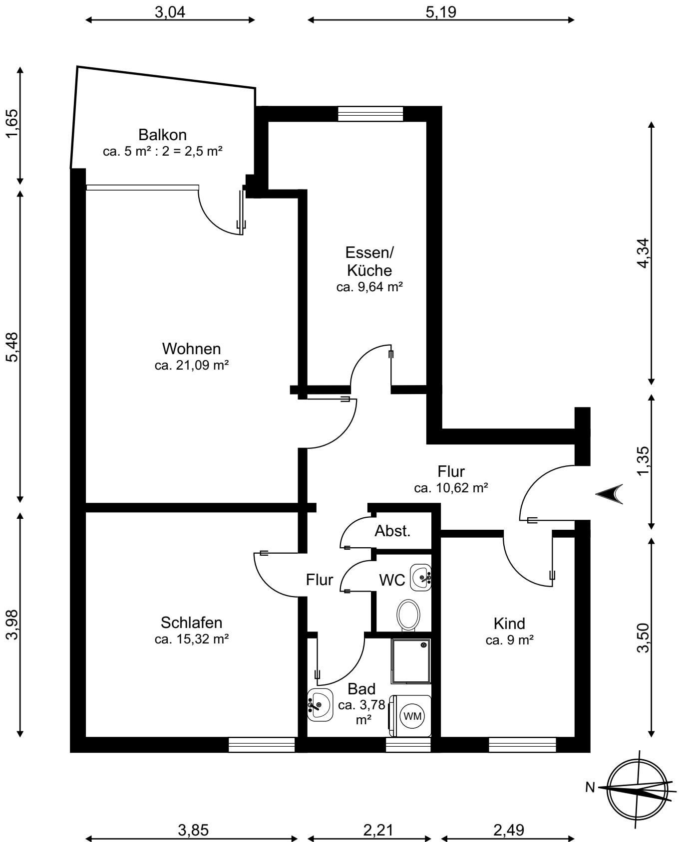
MB 24128 Grundriss
