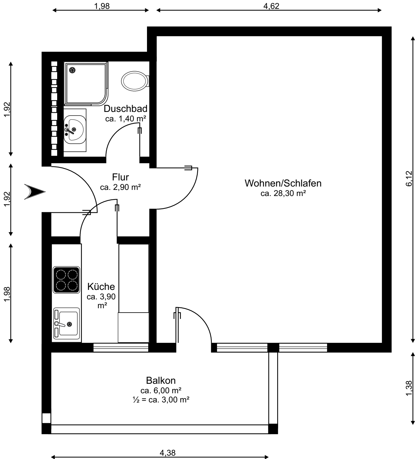
MK 25288 Grundriss 3.Obergeschoss
