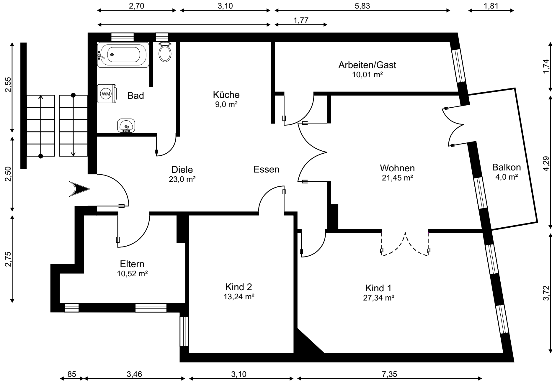
MB 23233 Grundriss
