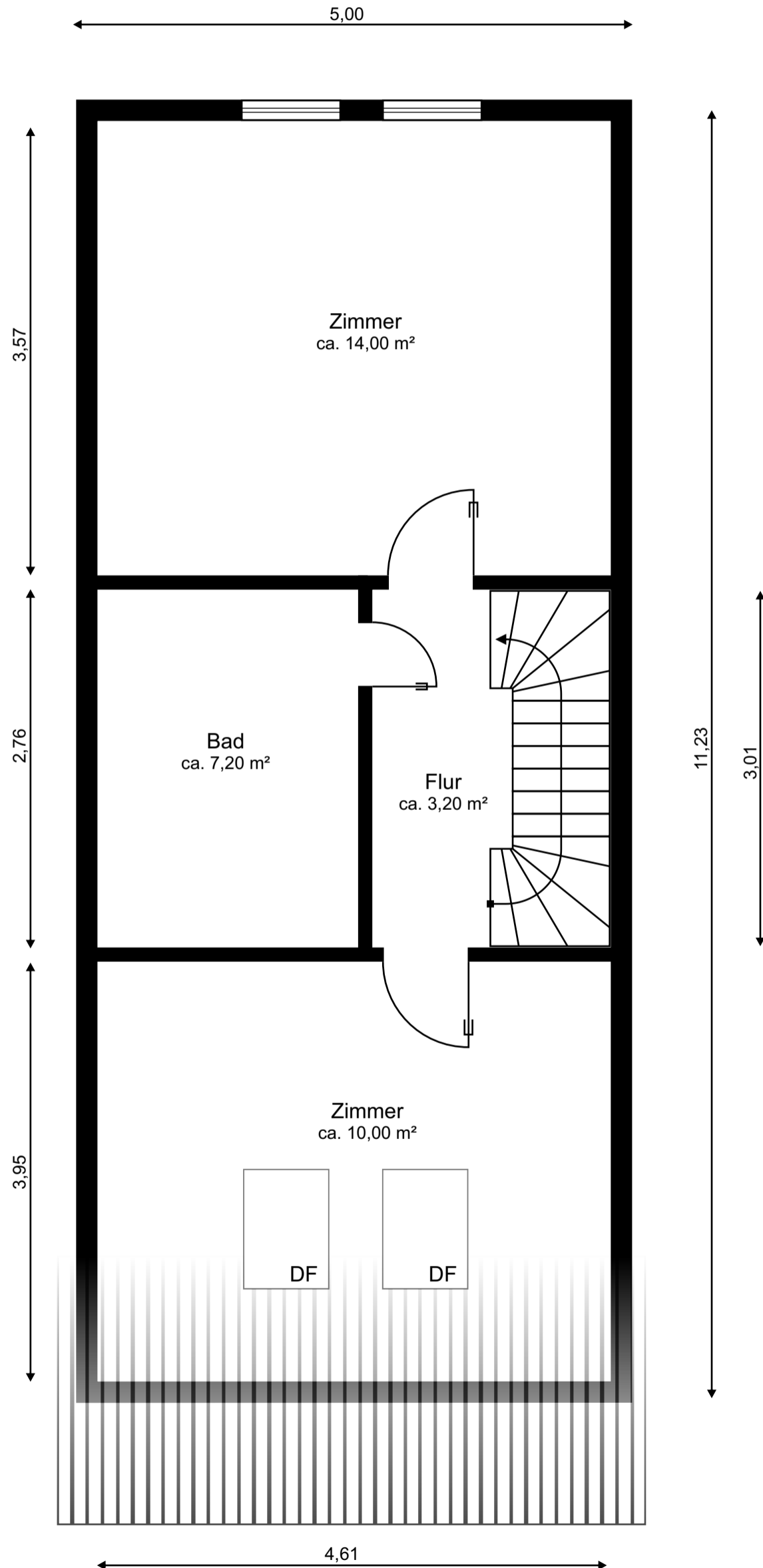
MB 24312 Grundriss Dachgeschoss
