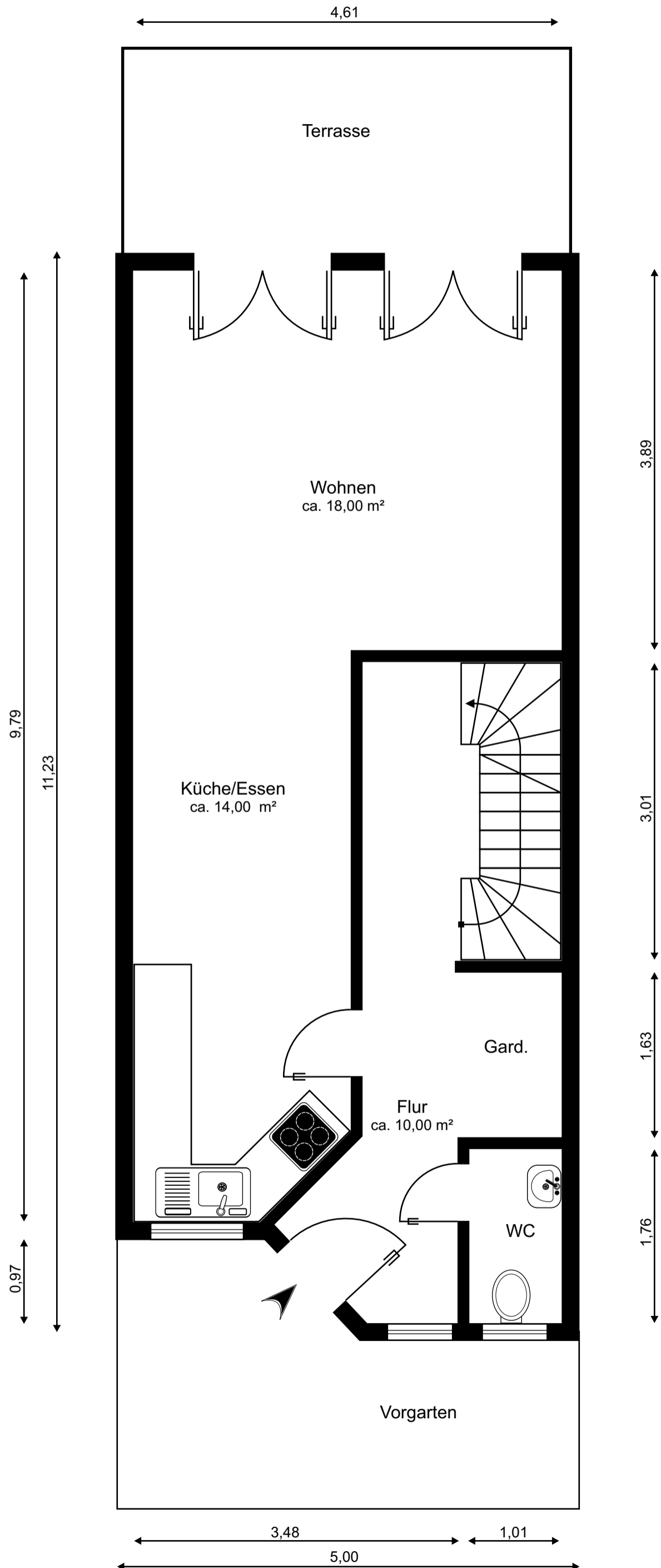
MB 24312 Grundriss Erdgeschoss
