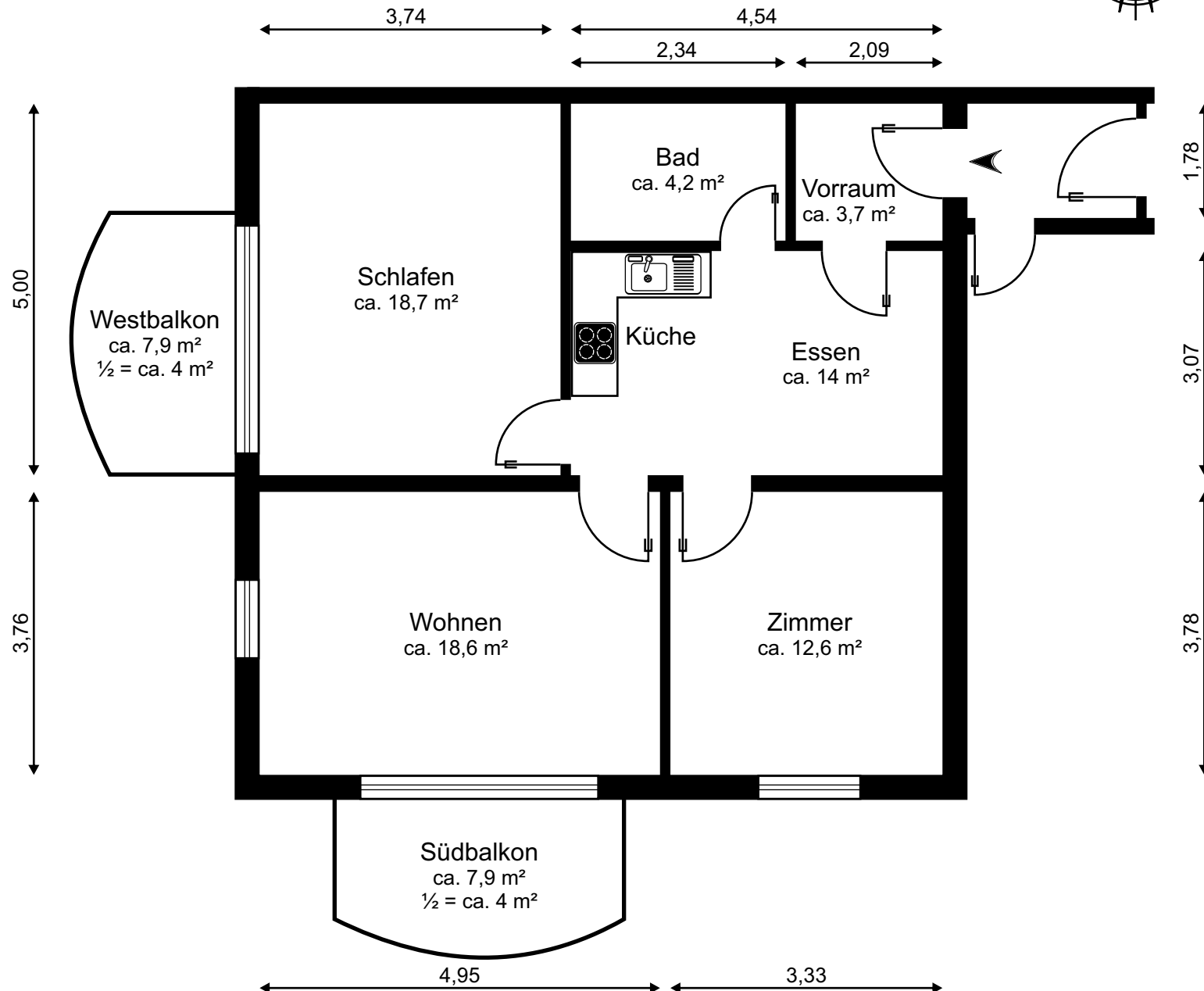
MB 25168 Grundriss
