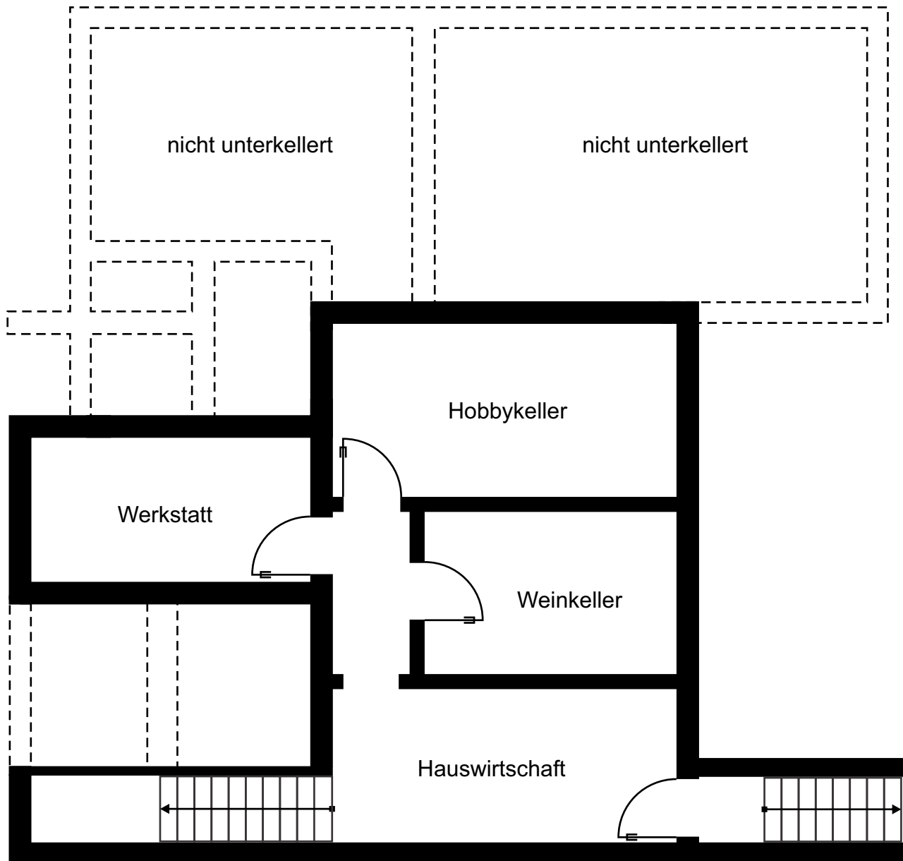
Grundriss Kellergeschoss MB 24186
