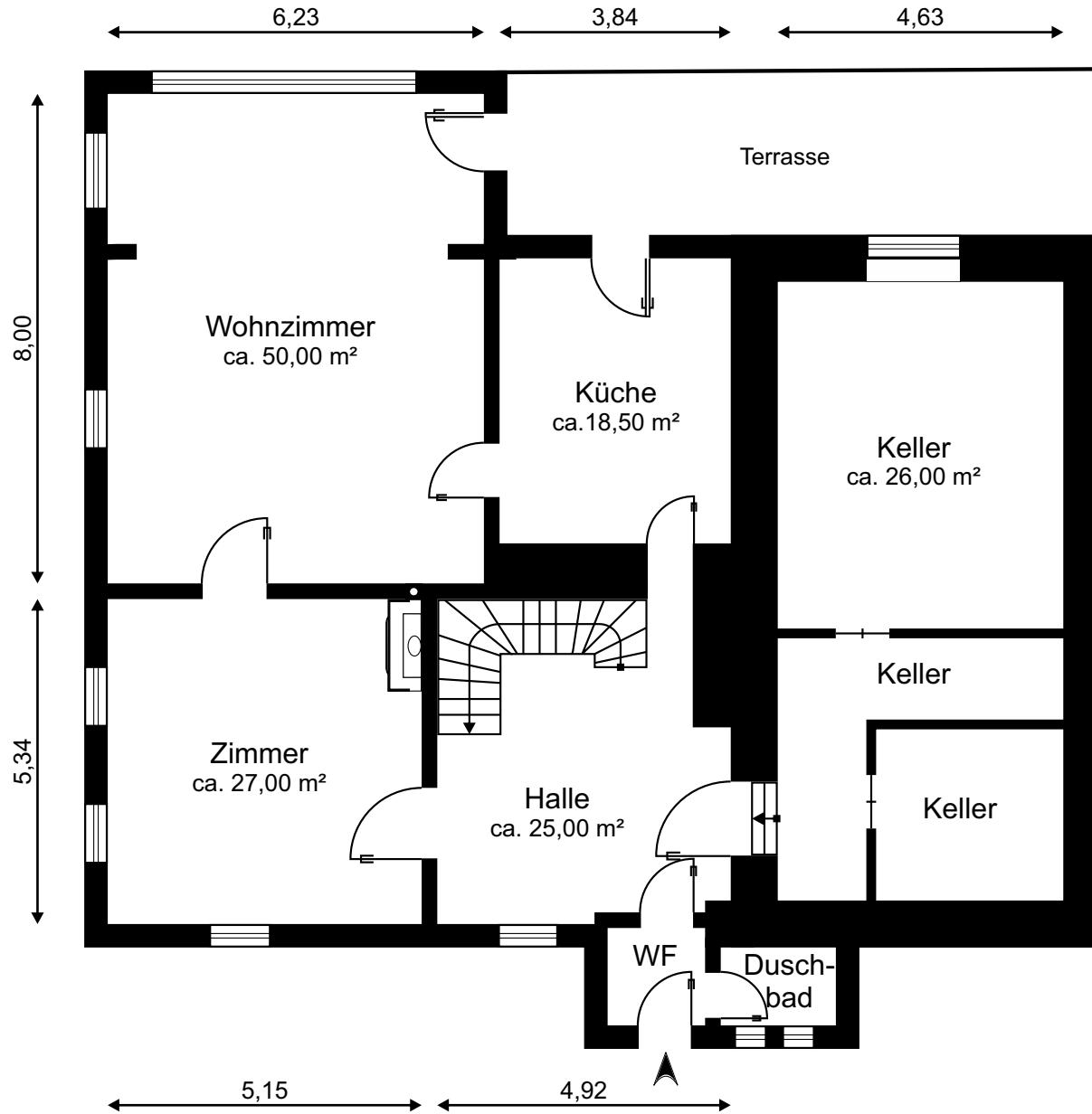
Erdgeschoss
