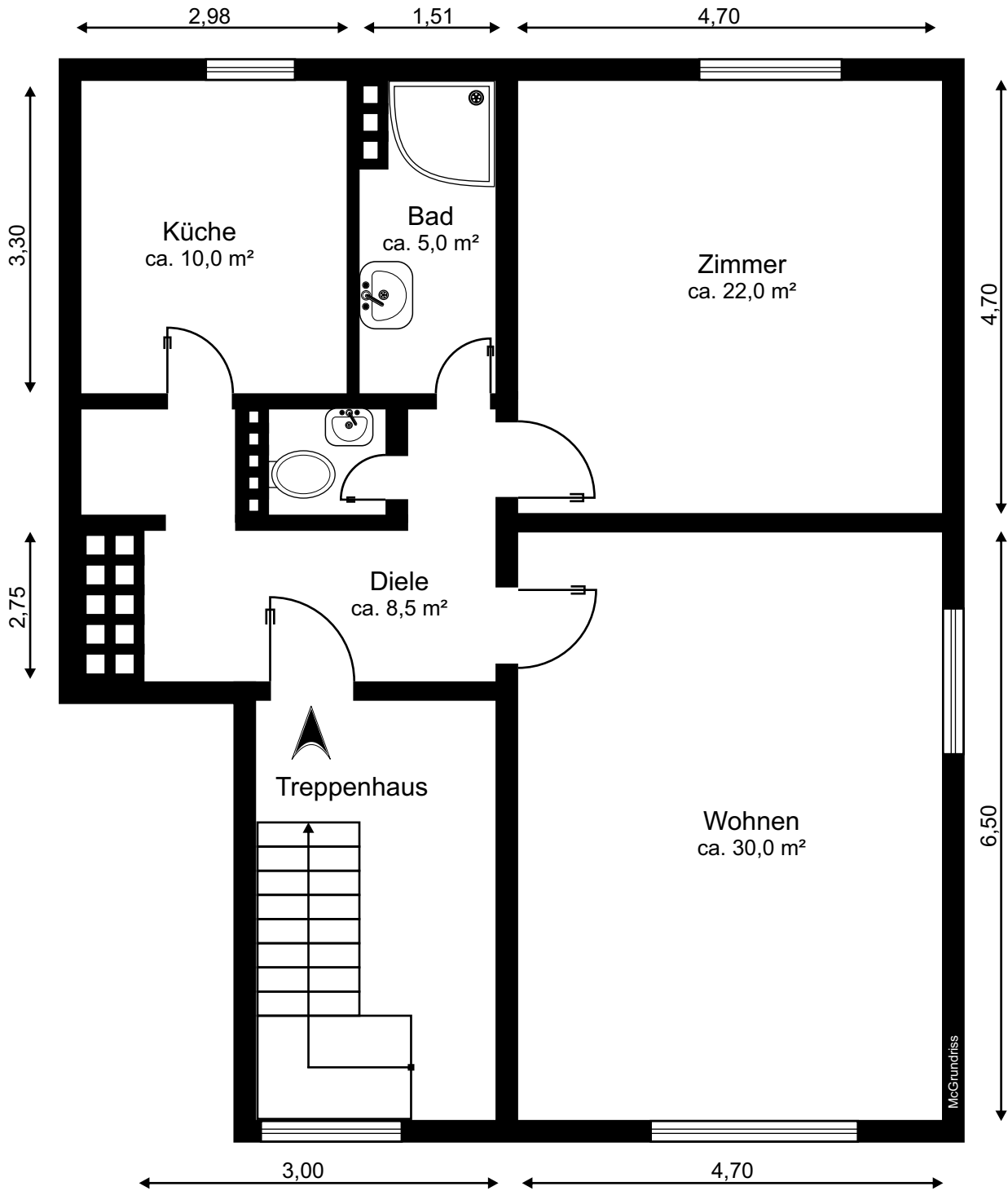
MB 25100 Grundriss
