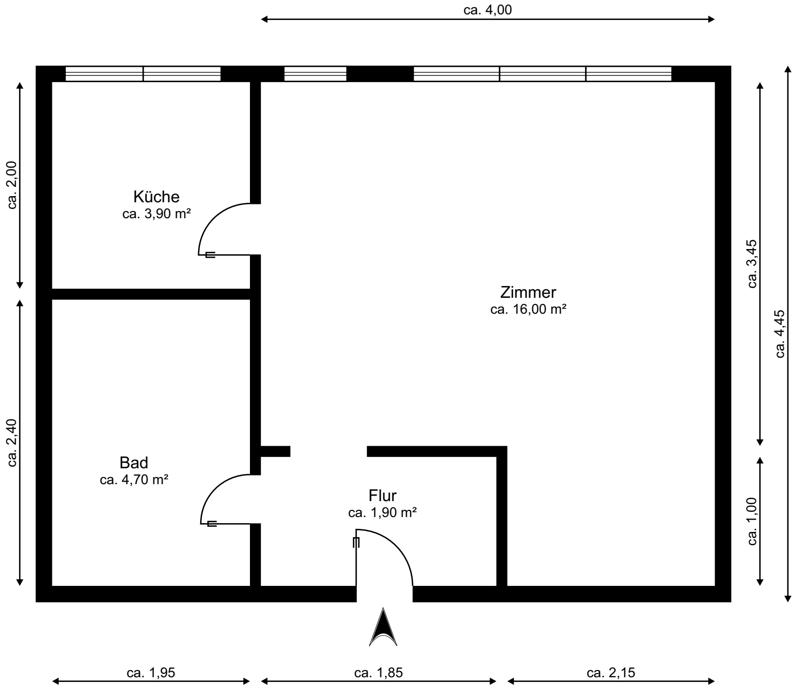
MK 20307 Grundriss
