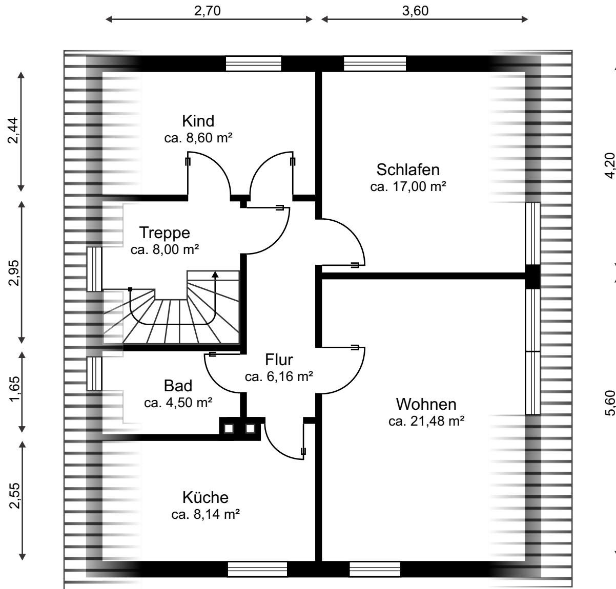
MB 22270 Grundriss Dachgeschoss
