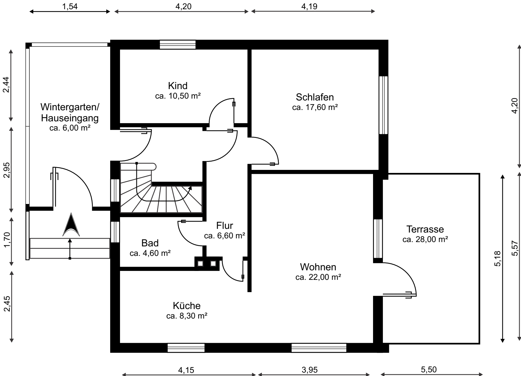
MB 22270 Grundriss Erdgeschoss
