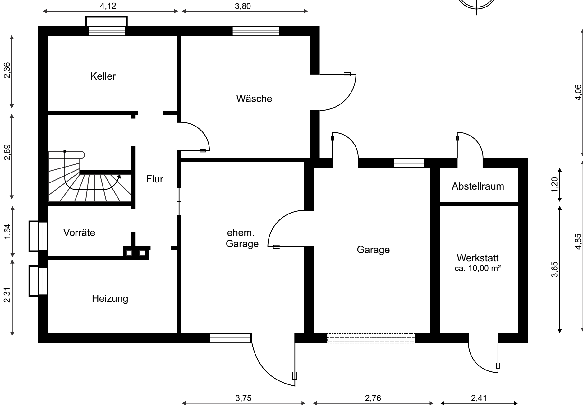
MB 22270 Grundriss Kellergeschoss
