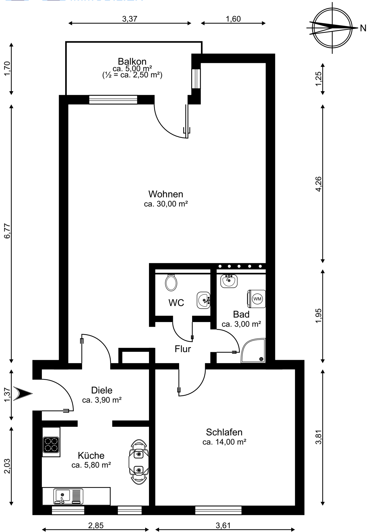
1. Obergeschoss
