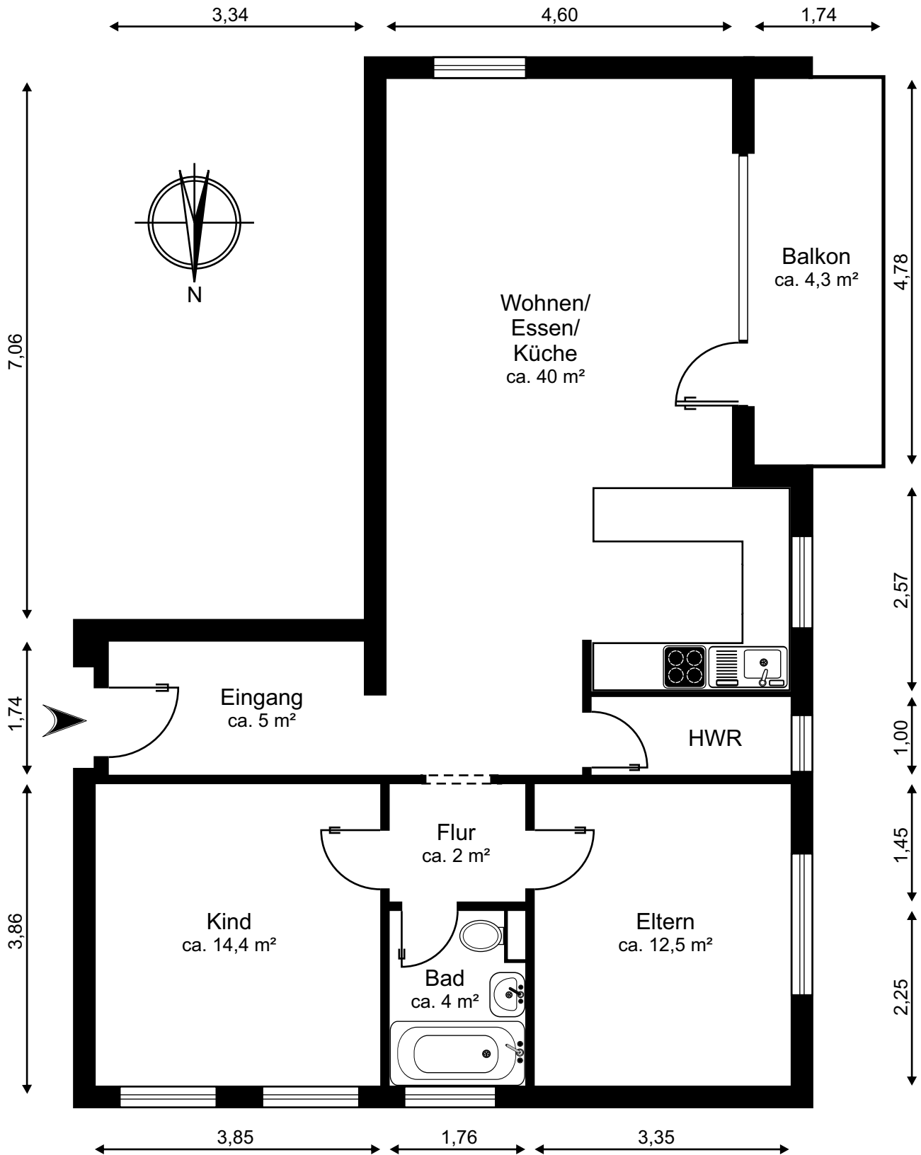
MB_23192 Grundriss
