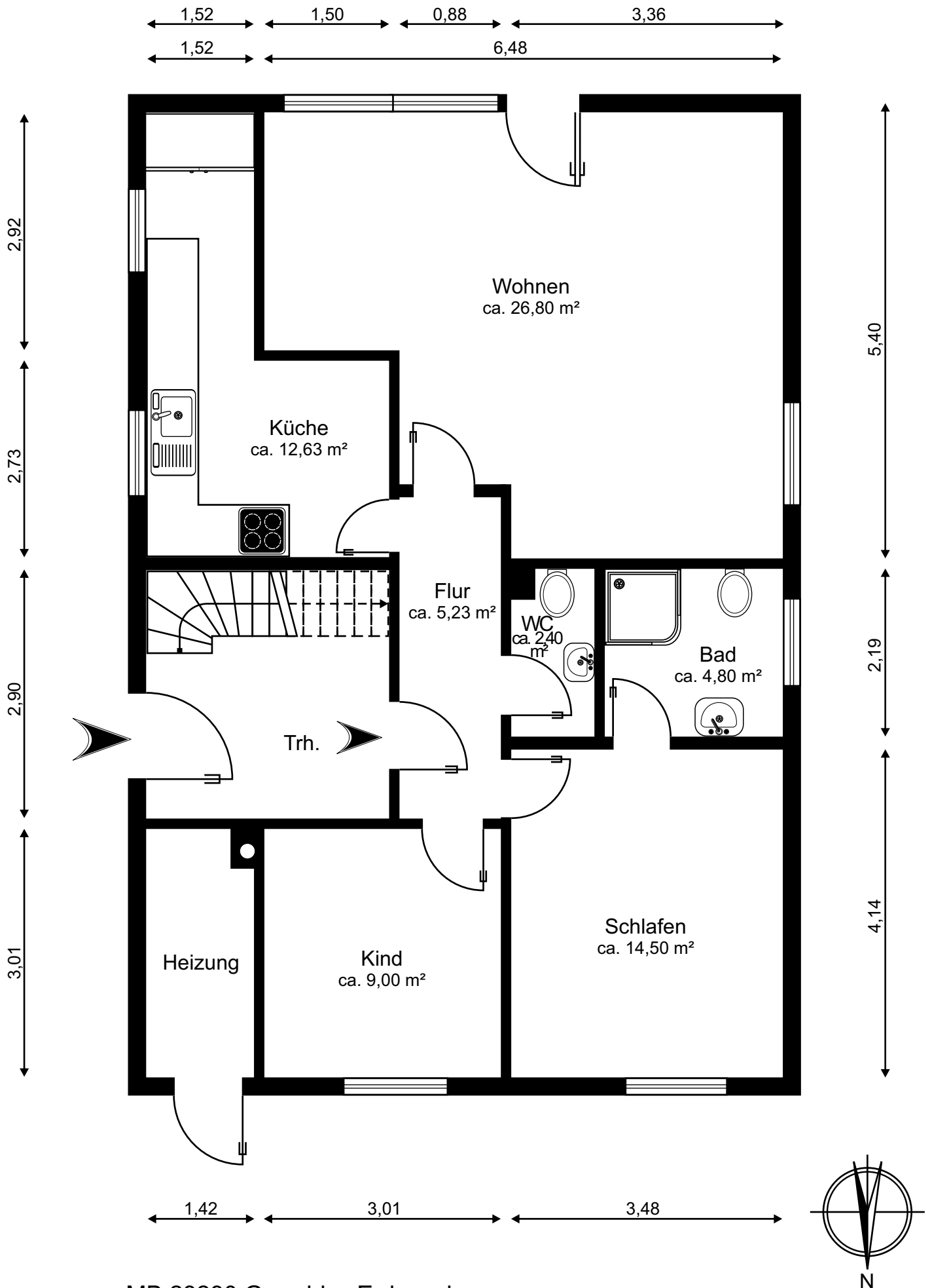
MB 23230 Grundriss Erdgeschoss
