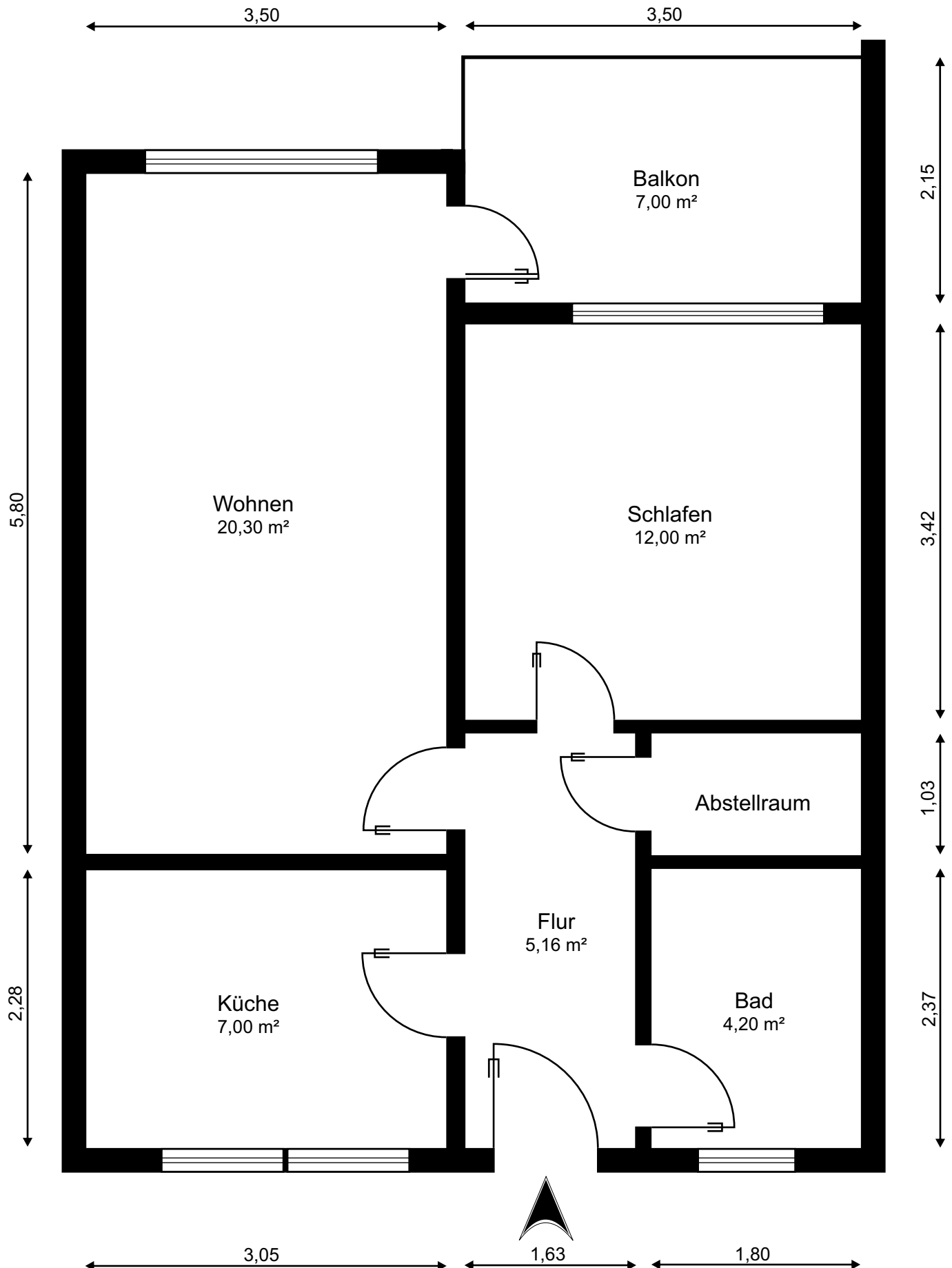
MB 25230 Grundriss
