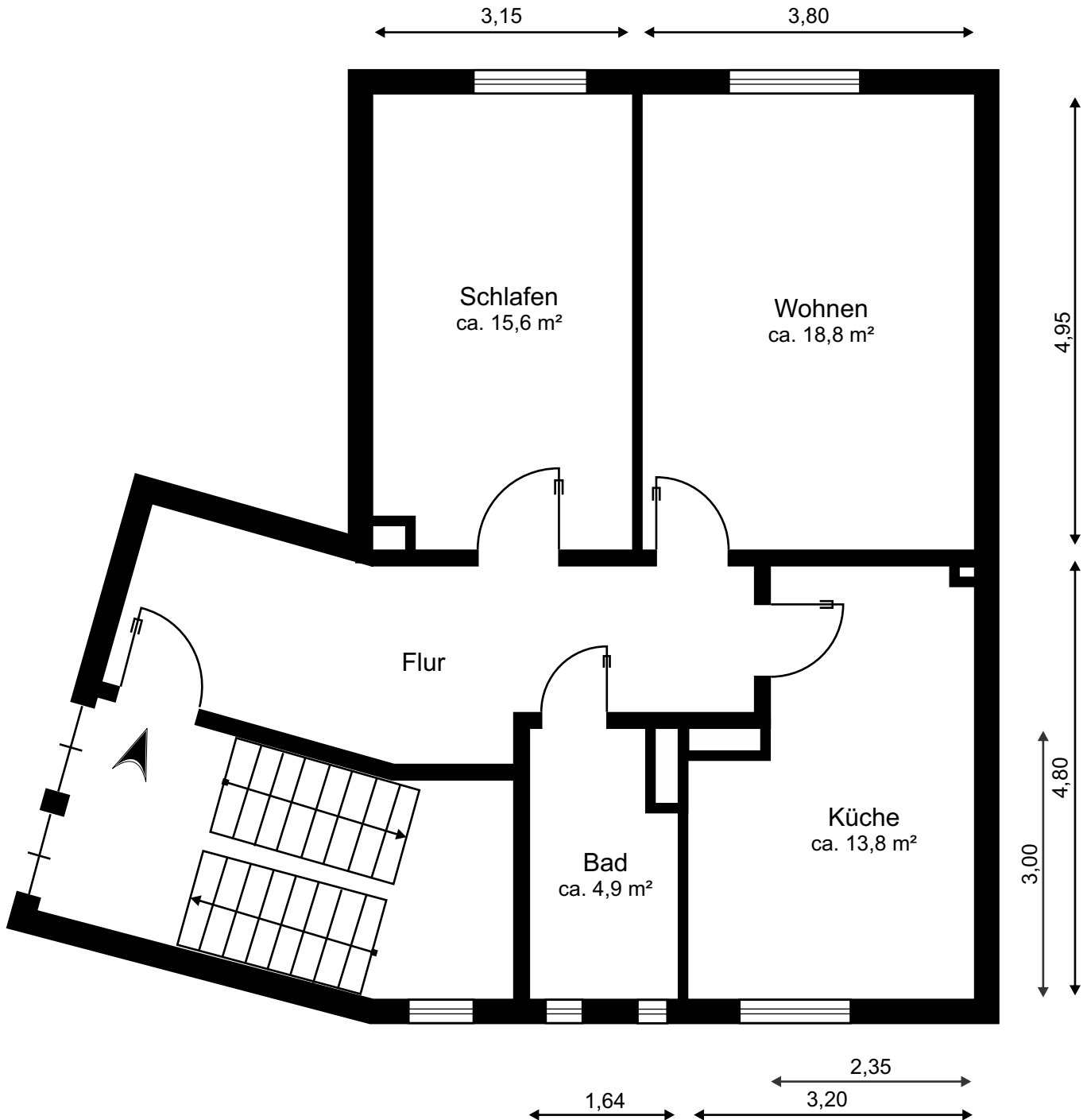
MK 22048 Grundriss
