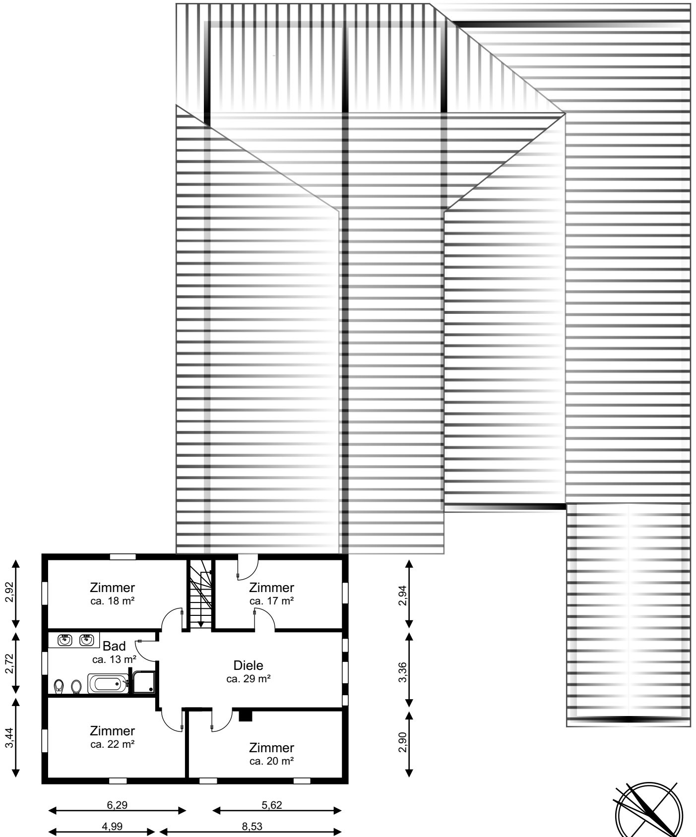
MB 20175 Grundriss
