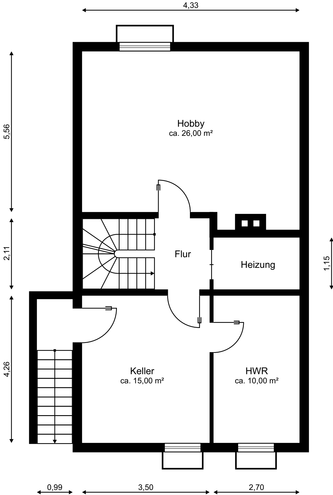
MB 23145 Grundriss Kellergeschoss
