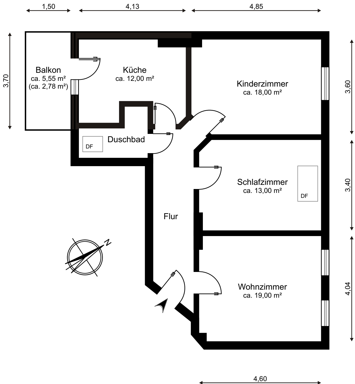
MB 17353 Grundriss
