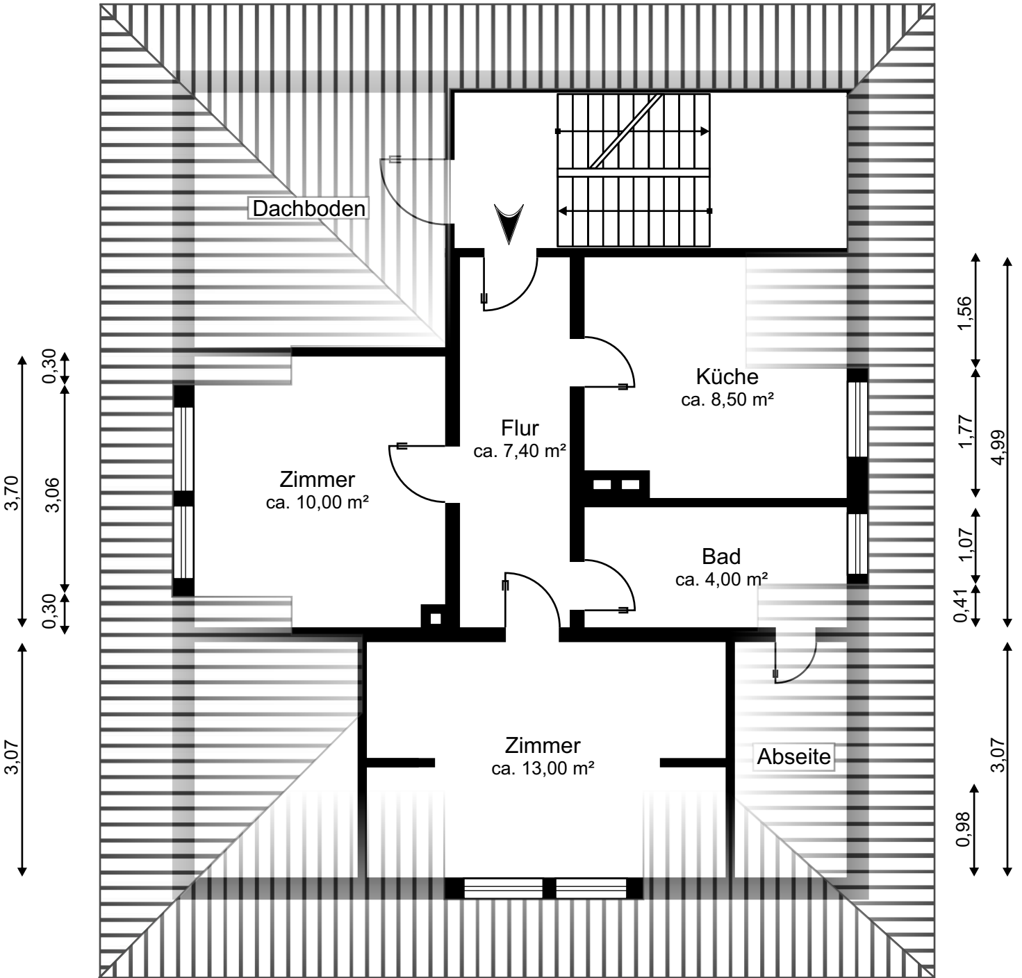
MK 19077 Grundriss DG
