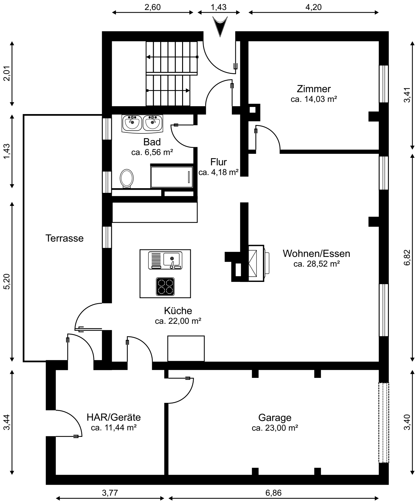
MB 26047 Grundriss Erdgeschoss
