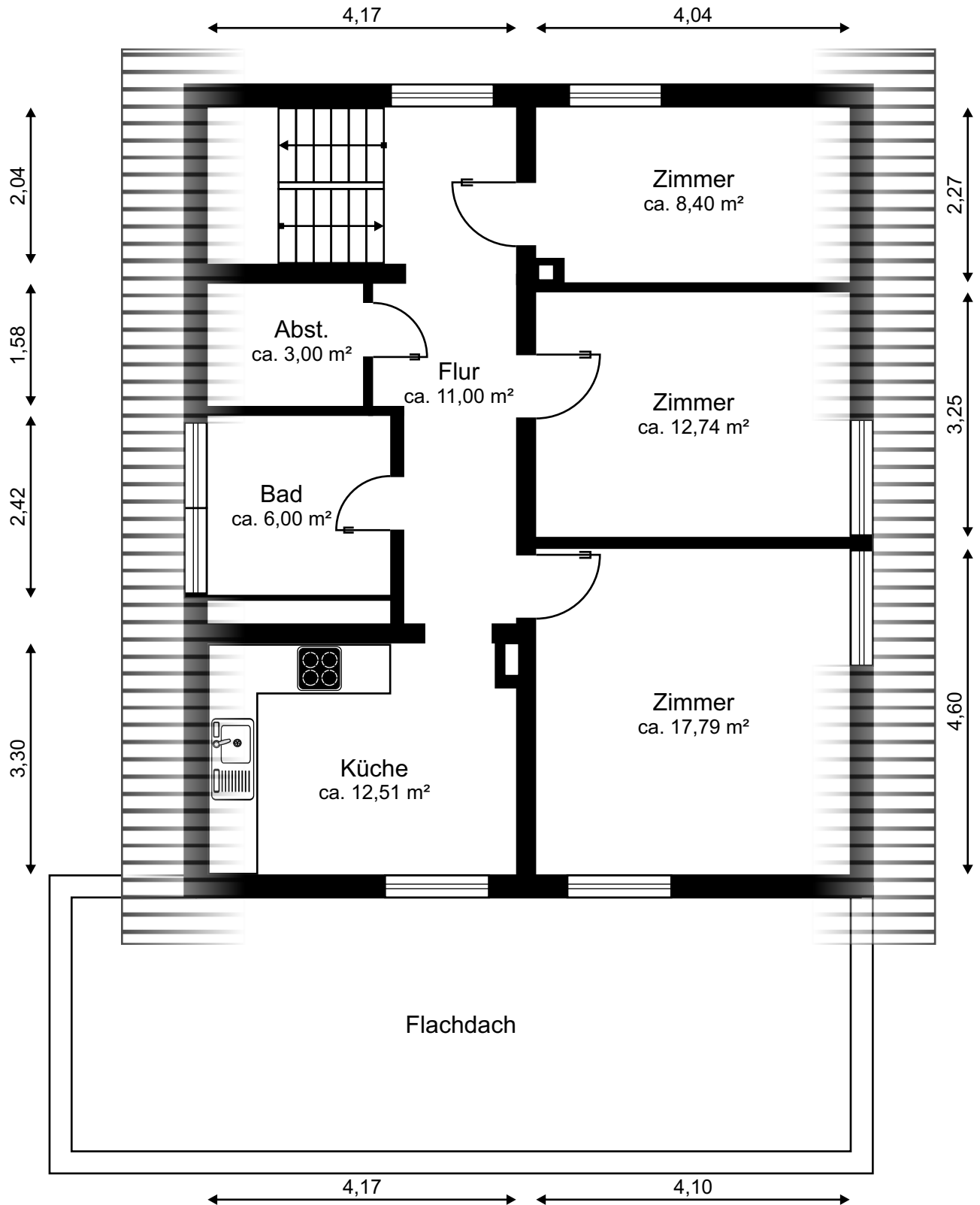
MB 26047 Grundriss Obergeschoss
