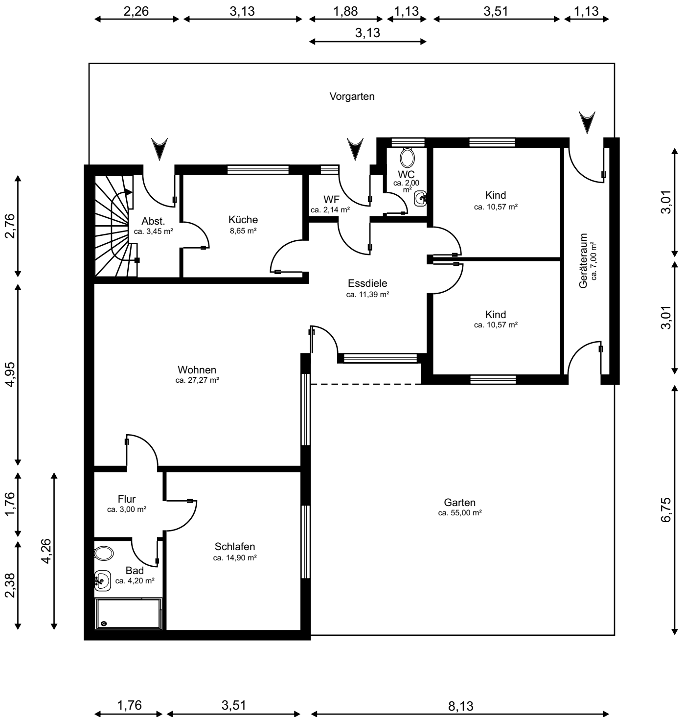
MB 26147 Grundriss Wohnen
