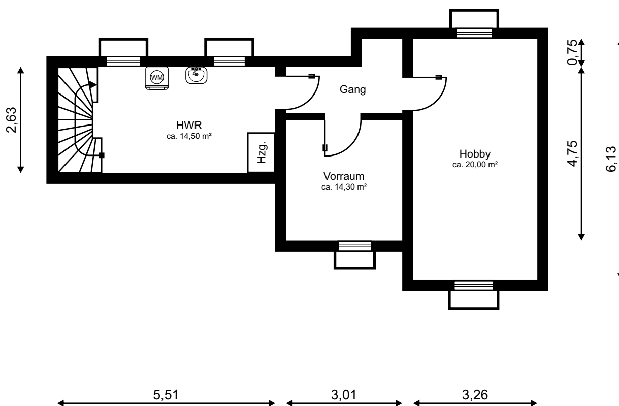
MB 26147 Grundriss Teilkeller
