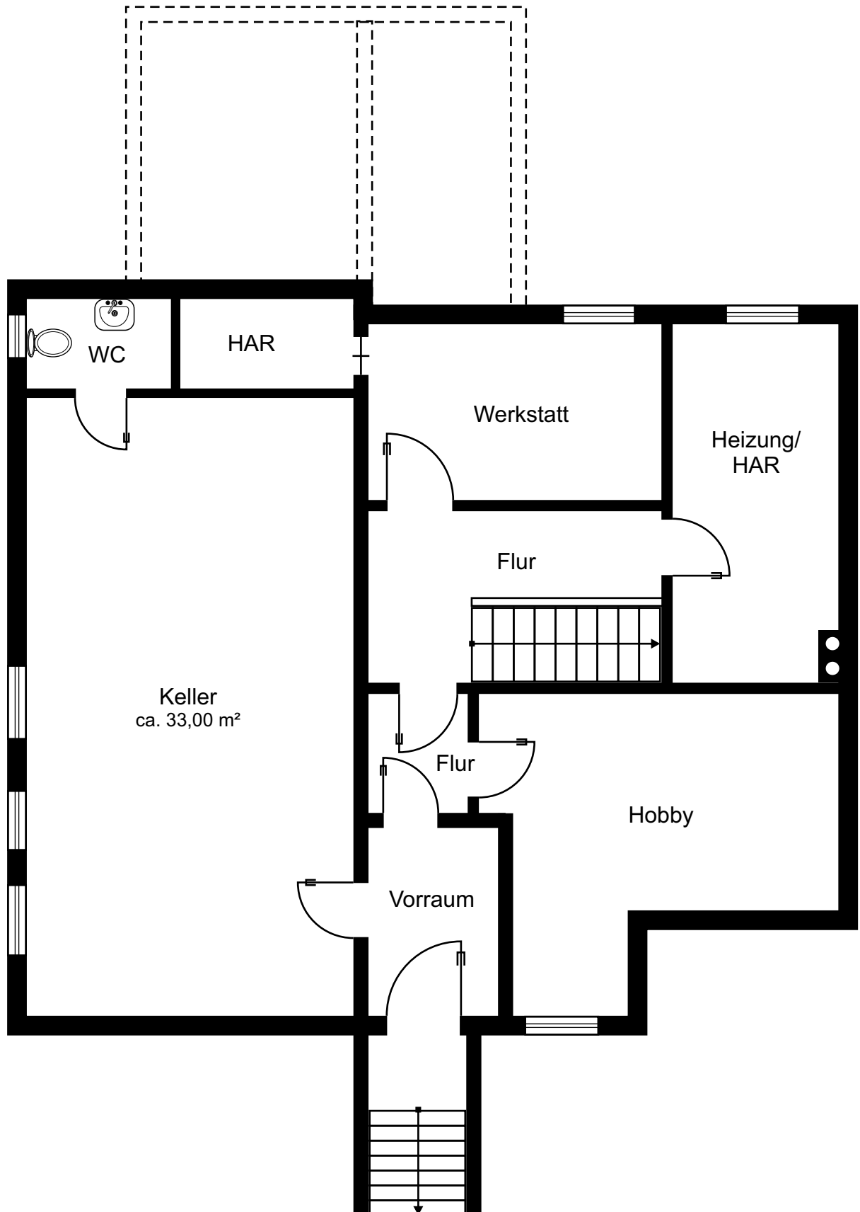
Kellergeschoss
