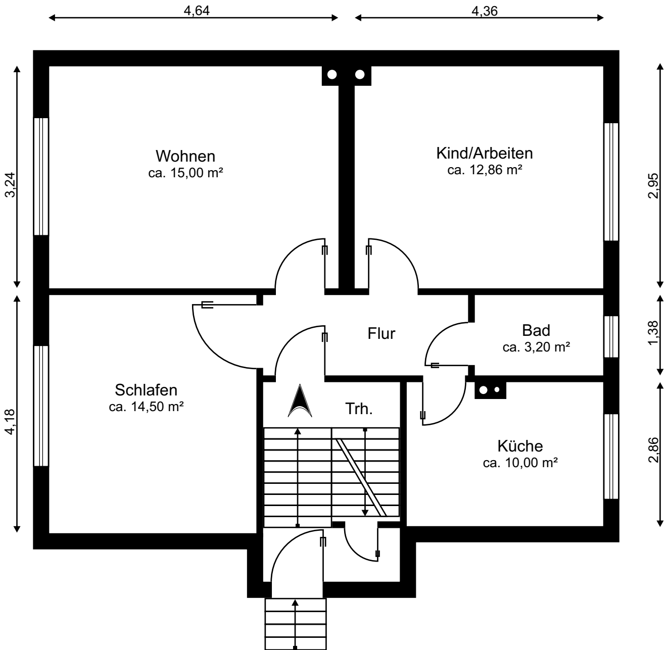
MB 24241 Grundriss Erdgeschoss
