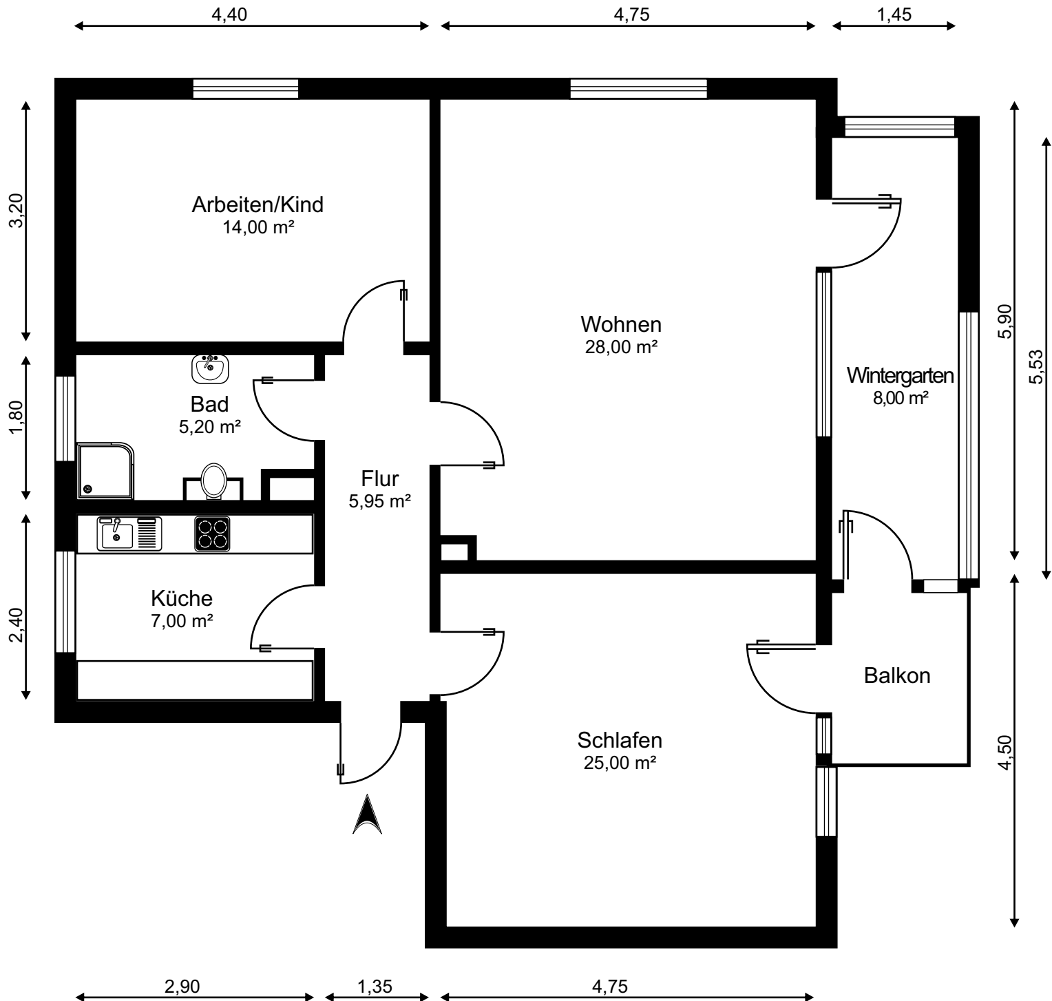
MK 25143 Grundriss
