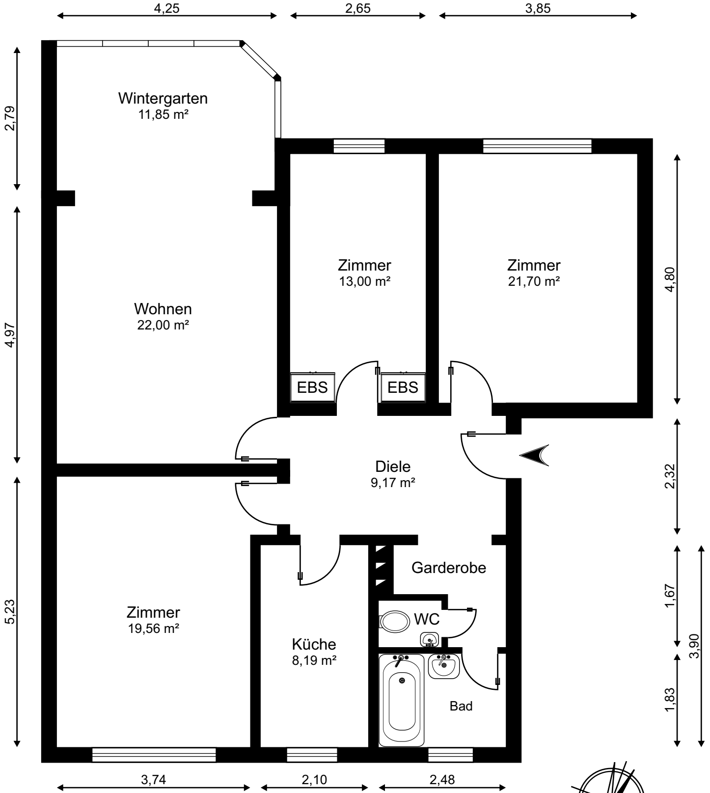
MK 23051 Grundriss 2.Obergeschoss
