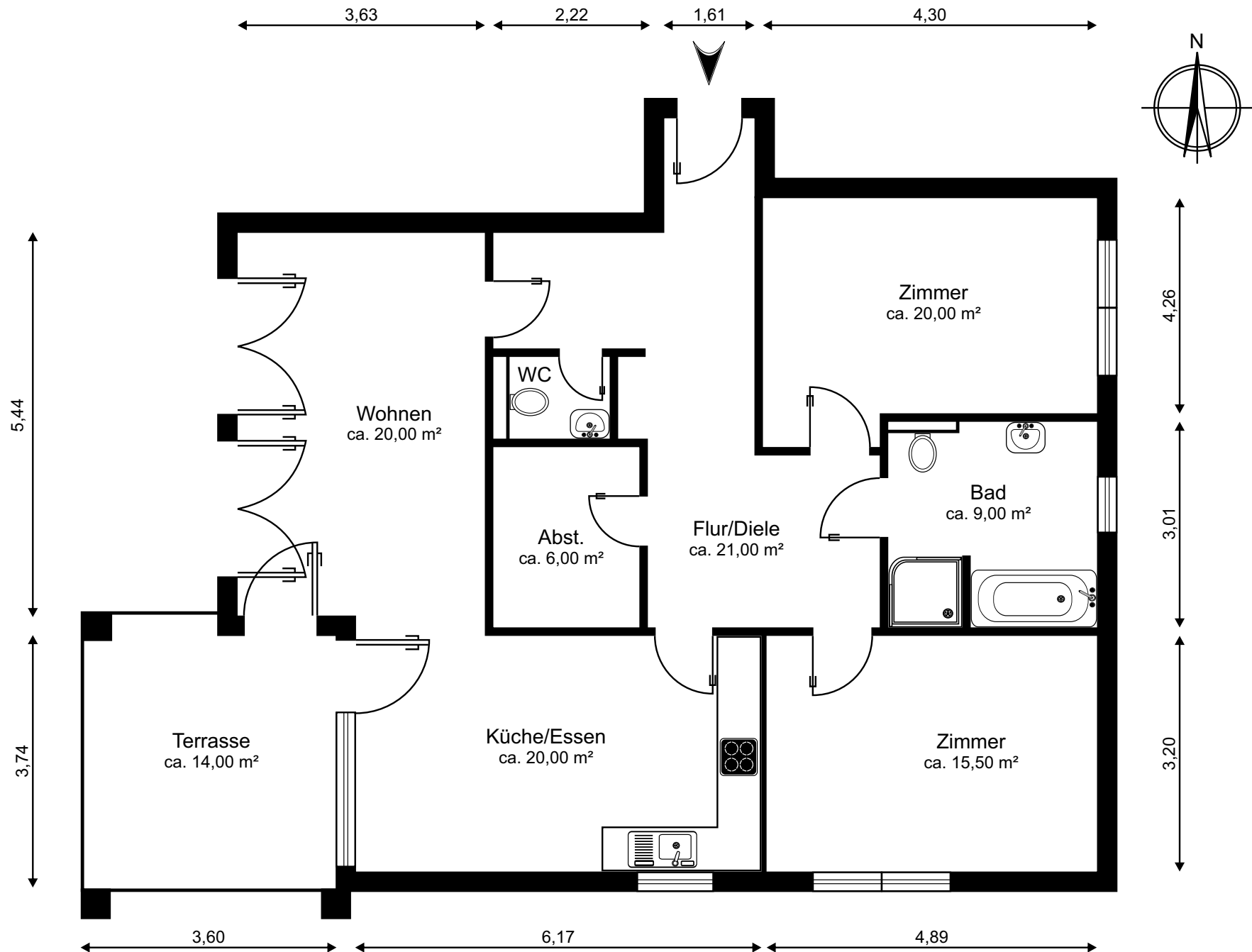
MK 21012 Grundriss
