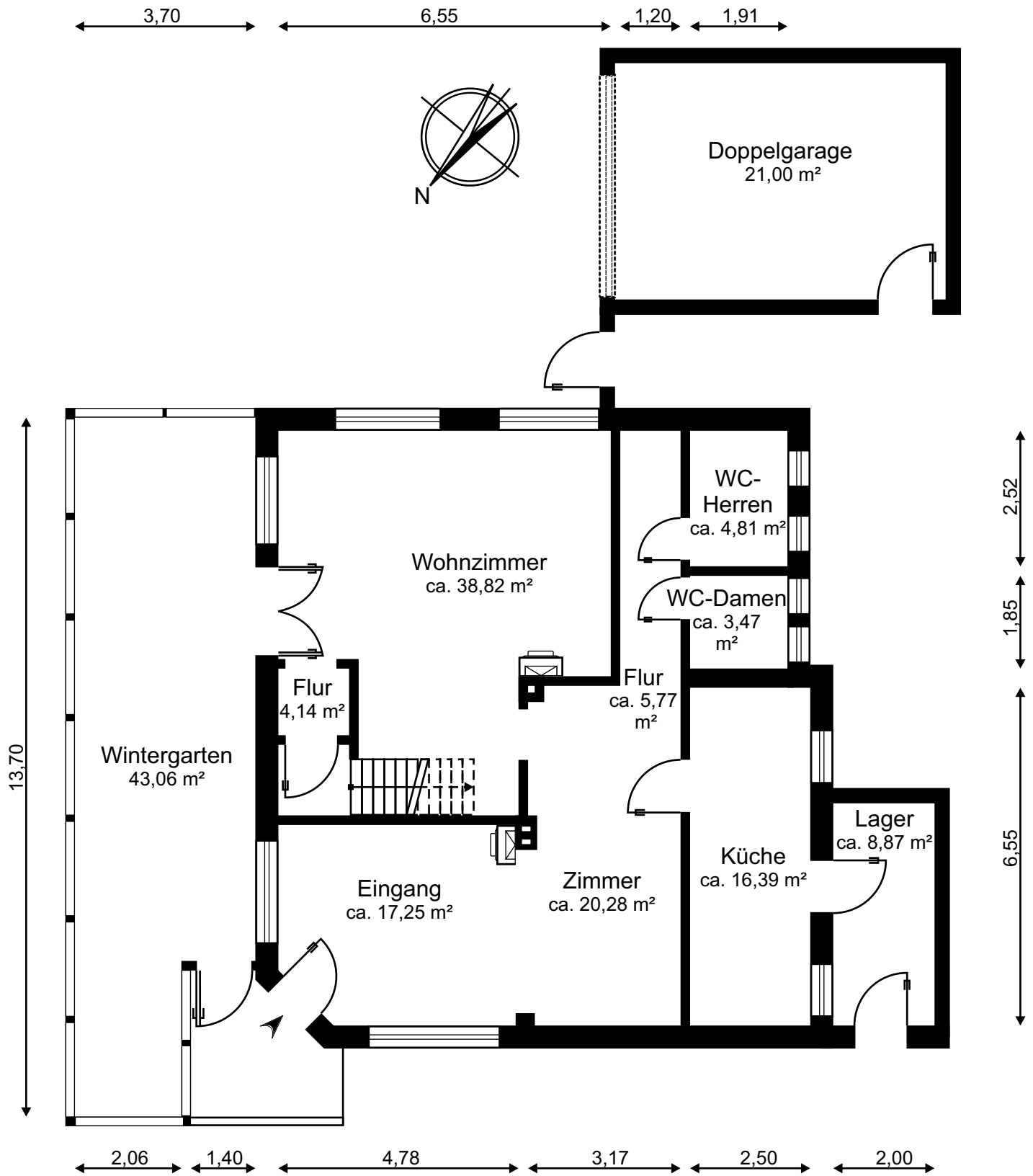
MB 24101 Grundriss Erdgeschoss
