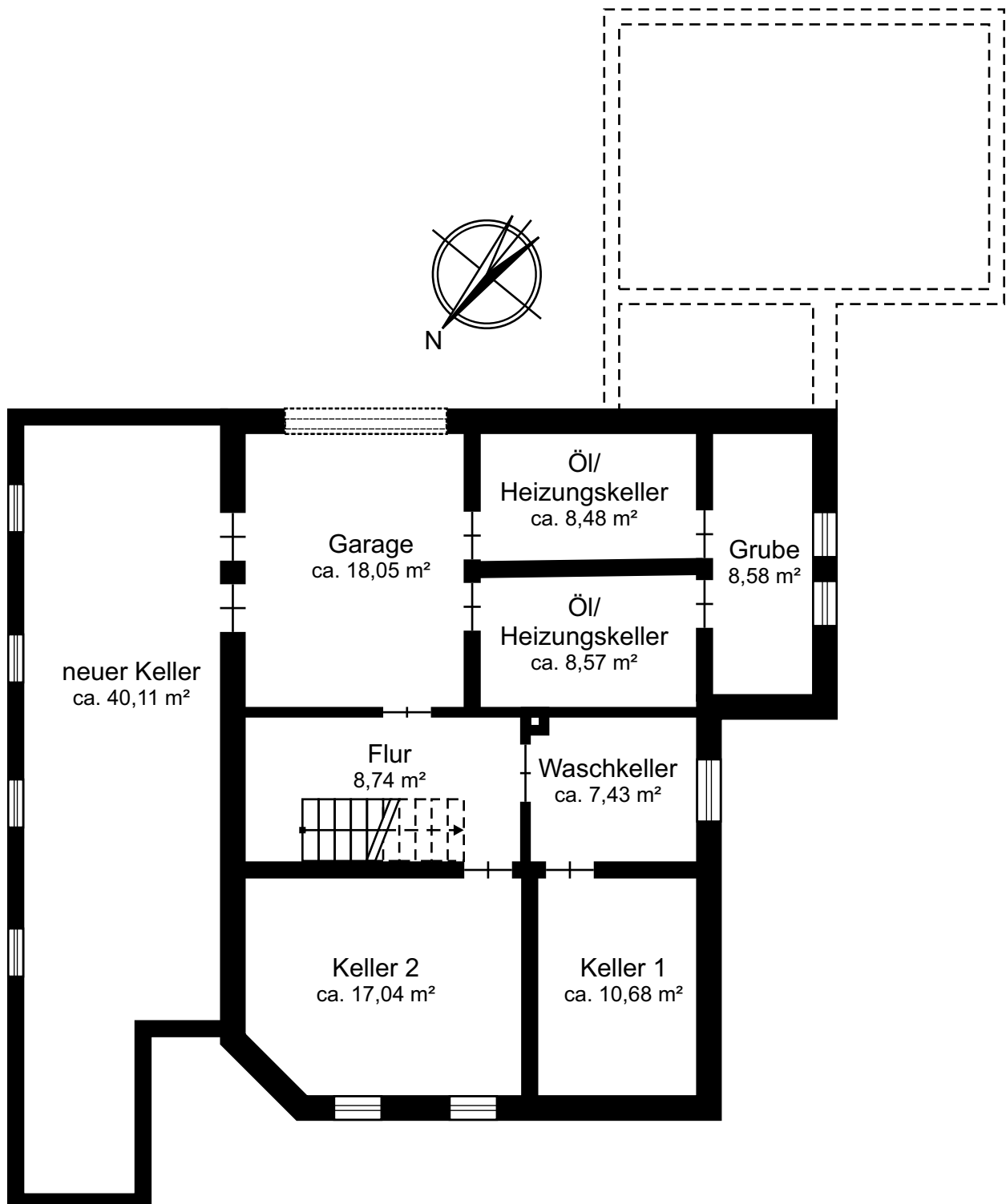
MB 24101 Grundriss Kellergeschoss
