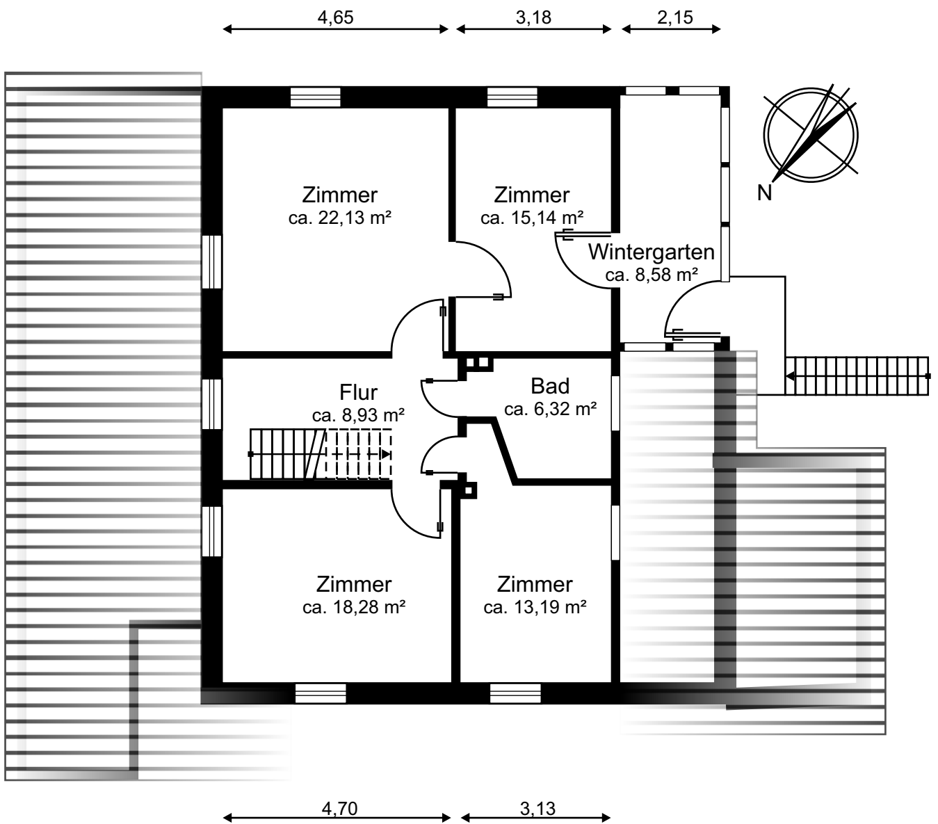
MB 24101 Grundriss Obergeschoss
